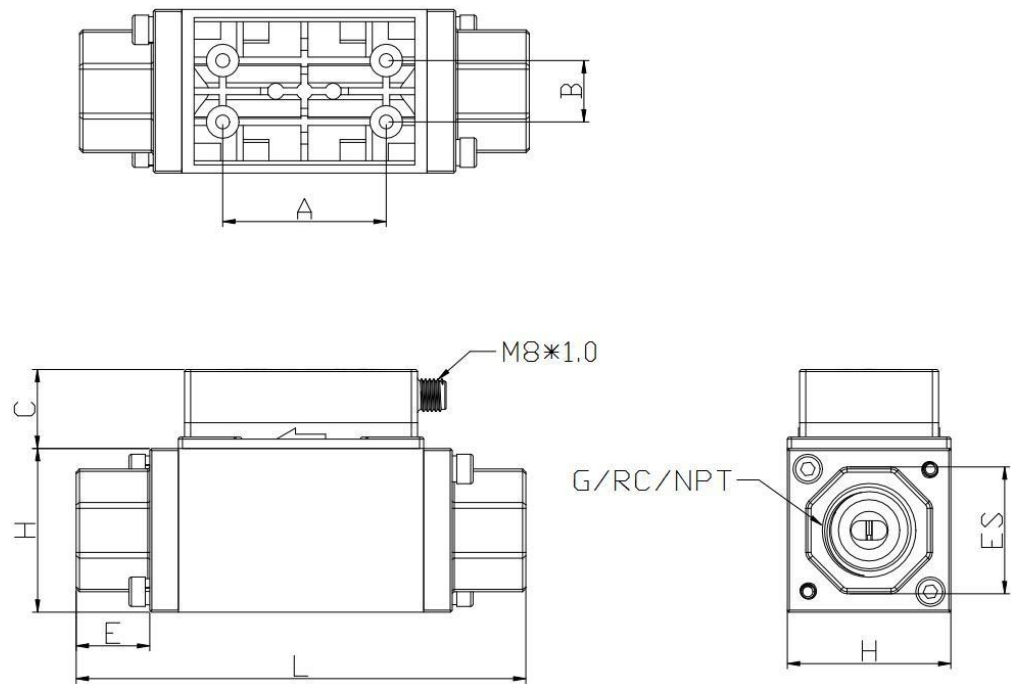
图7. MS-FX40系列外形尺寸图（单位：mm，L公差：±1mm,其余未标公差：±0.5
