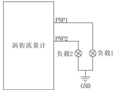
图 6. PNP 输出典型电路
