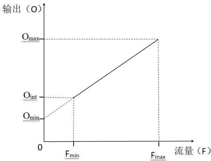
图 4. MS-FX40 系列流量与输出的对应线性图
