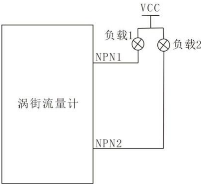
图 5. NPN 输出典型电路图
